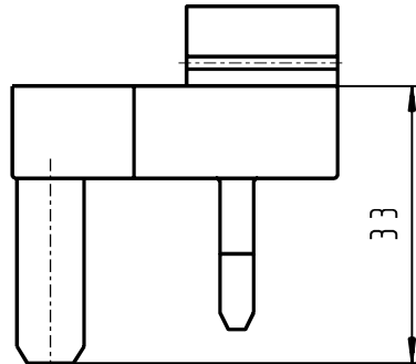
UK-Stecker 1717618 UK-plug 1717618
